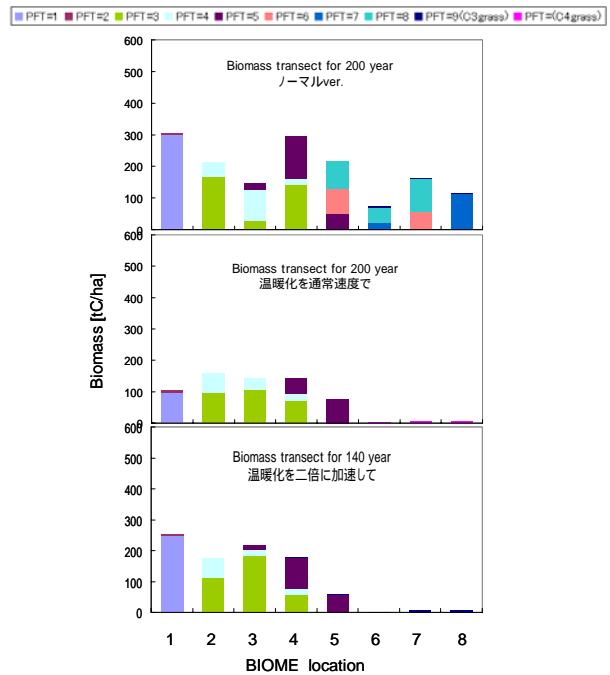
Fig.7：通常的气候(上図)、温暖化(中央図)、温暖化を加速(下図)の条件で計算したモデルのバイオマス量変化
